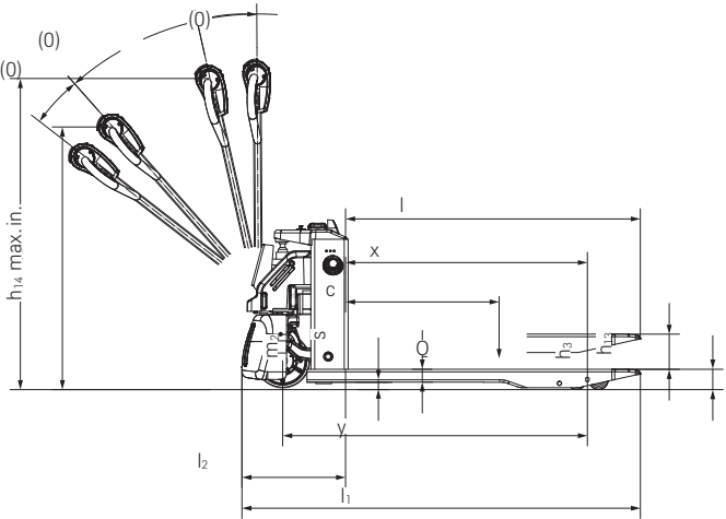
ECH 12C/15C zijaanzicht
