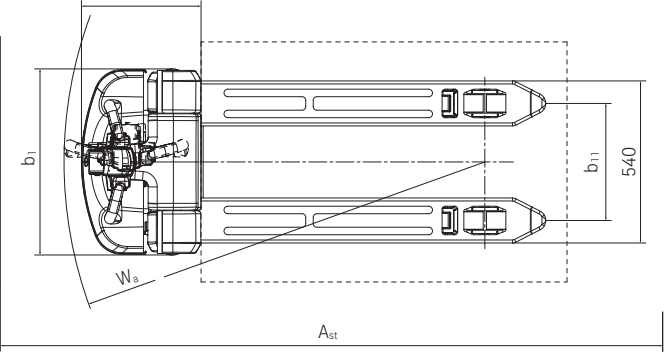
ECH 15 bovenaanzicht
