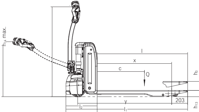
ECH 15 zijaanzicht
