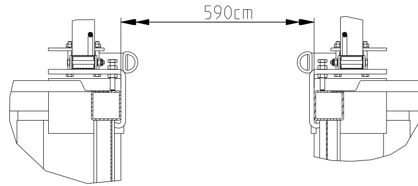
Schnitt / SECTION / doorsnede A-A
